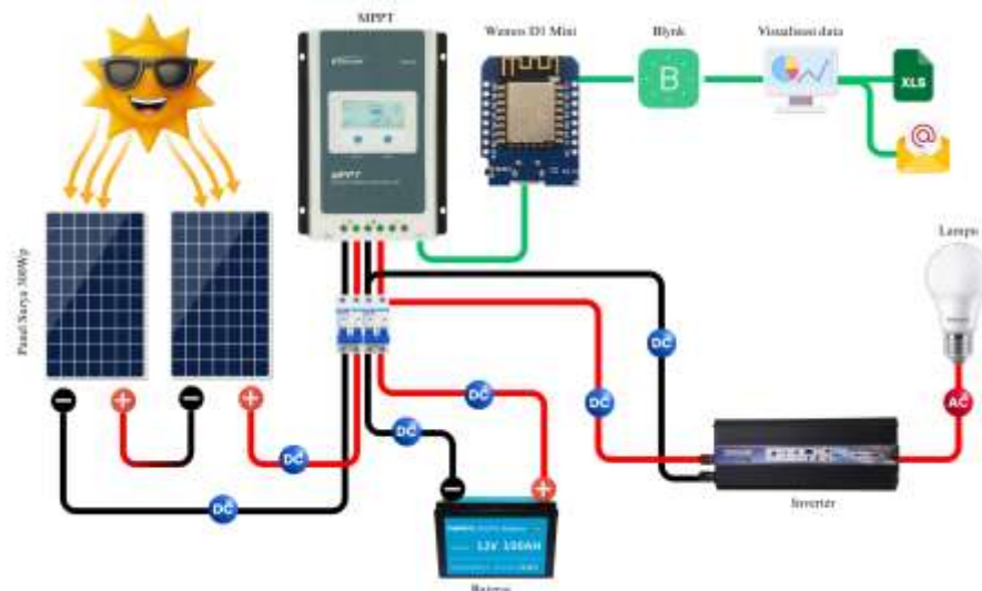
Gambar 3. Arsitektur sistem secara keseluruhan.
