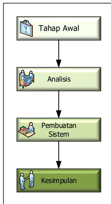
Gambar 1. Tahapan Penelitian
