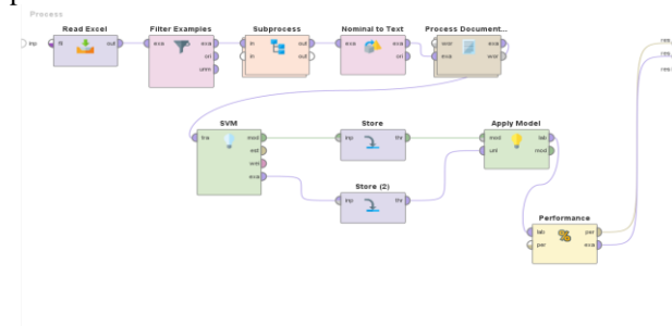
Gambar 10. Pembuatan Model Support Vector Machine
