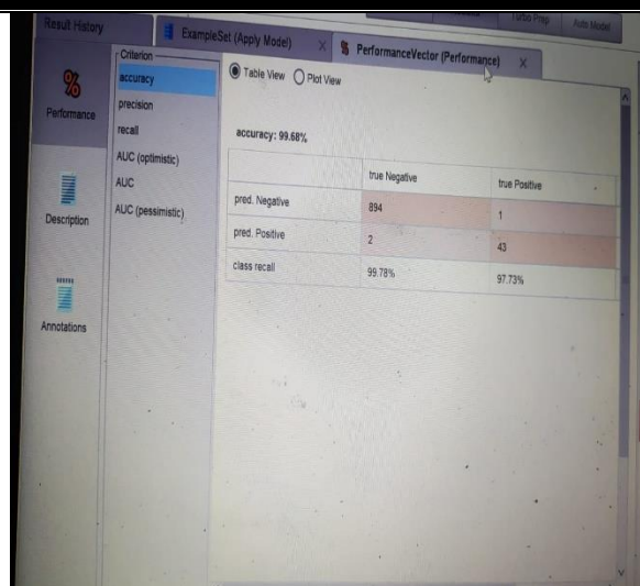
Gambar 15. Hasil Pengujian Naive Bayes
