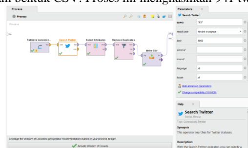
Gambar 2. Proses Pengumpulan Data
