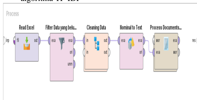
Gambar 12. Pembuatan Model Support Vector Machine
